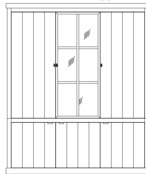
VITRINE 3M - 2 DOORS WOOD + 1 DOOR METAL 1840 x 480 x 2190(H)
