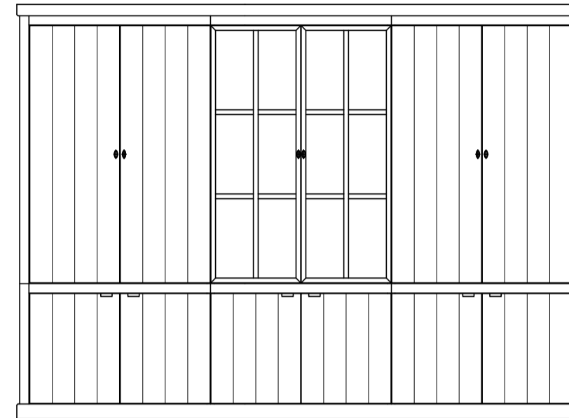
VITRINE 6M - 2 DOORS METAL + 4 DOOR WOOD 3000 x 480 x 2190(H)
