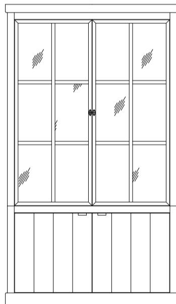
VITRINE 2Y - 2 DOORS METAL 1271 x 480 x 2190(H)
